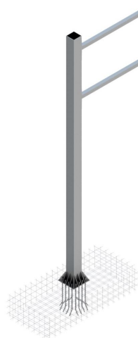
Galgpaal
